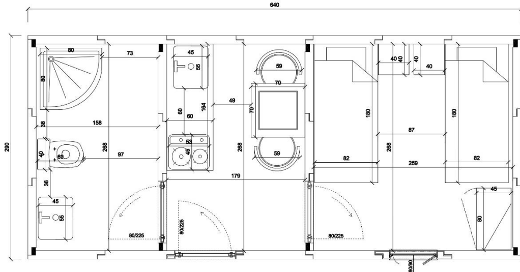
Şekil 5.12. 3 modülden oluşan Modüler konut planı (Kişisel Arşiv).
