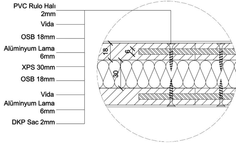
Şekil 5.9. Döşeme detayı (Kişisel Arşiv).
