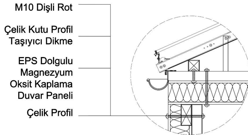
Şekil 5.10. Çatı, oluk ve duvar paneli bağlantı detayı (Kişisel Arşiv).
