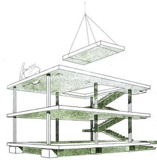
Şekil 4.8. Domino Evi inşa görselleştirmesi(Url 21).
