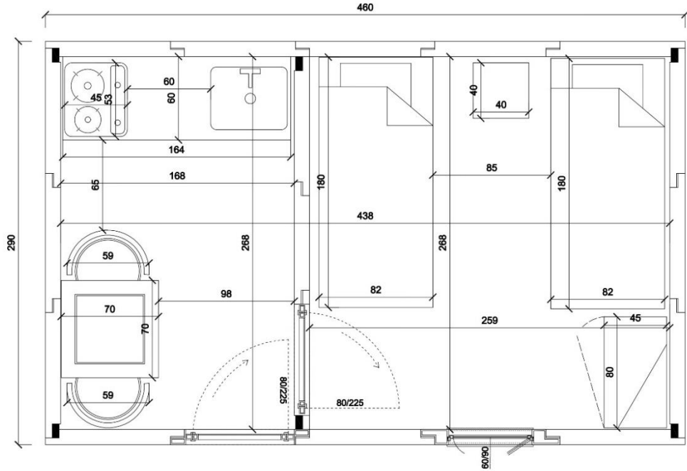
Şekil 5.13. 2 modülden oluşan Modüler konut planı (Kişisel Arşiv).
