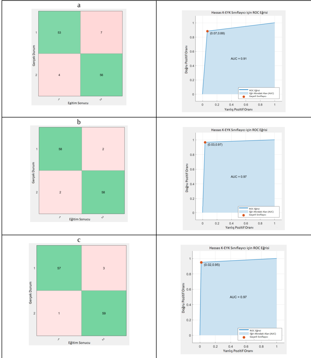
Şekil 4.1. Hassas K-EYK modelinin ünlü (a), ünsüz (b) ve tüm sesler (c) için eğitim sonuçlarına ait hata matrisleri ve ROC eğrileri.
