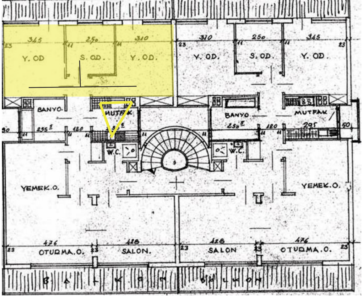
Şekil 5.41. 1955 Kütüphane Evleri Normal Kat Planı. Kaynak: Sivil Mimari Bellek Ankara 1930-1980
