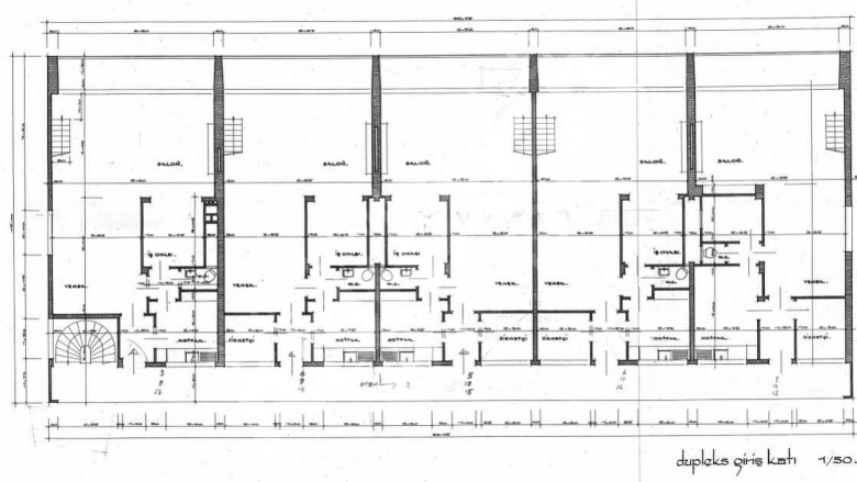
Şekil 4.26. Cinnah 19 Plan, URL 15 Erişim: 18.05.2025
