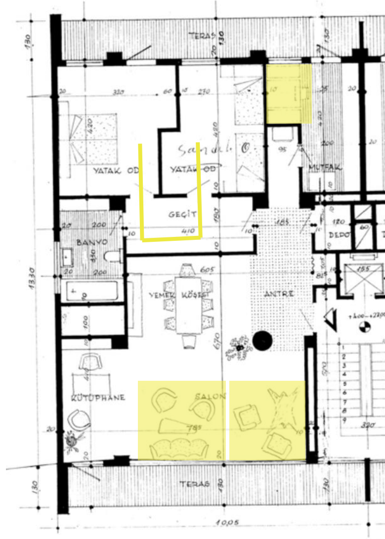
Şekil 5.43. 1957 Mintrak Apartmanı, Normal Kat Planı. Kaynak: Sivil Mimari Bellek Ankara 1930-1980 Projesi Arşivi, URL 22 Erişim:03.05.2025
