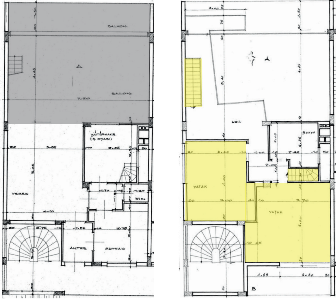
Şekil 5.49. 1958 Cinnah 19 Apartmanı, Dubleks Konut Giriş ve Üst Kat. Kaynak: Sivil Mimari Bellek Ankara 1930-1980 Projesi Arşivi, URL 22 Erişim:03.05.2025
