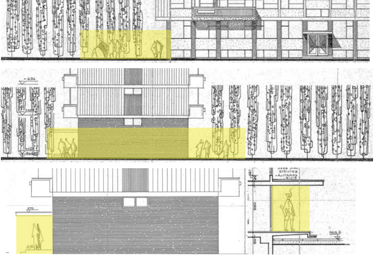
Şekil 5.96. 1959 İmar Blokları Mimari Çizimler. Kaynak: Sivil Mimari Bellek Ankara 1930-1980 Projesi Arşivi, URL 22 Erişim:03.05.2025
