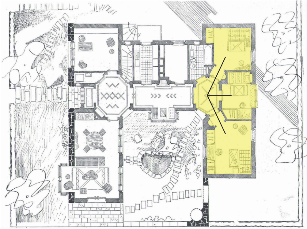
Şekil 5.35. 1952 Ekrem Baydar Evi Vaziyet Planı. Kaynak: Sivil Mimari Bellek Ankara 1930-1980 Projesi Arşivi, URL 22 Erişim:03.05.2025
