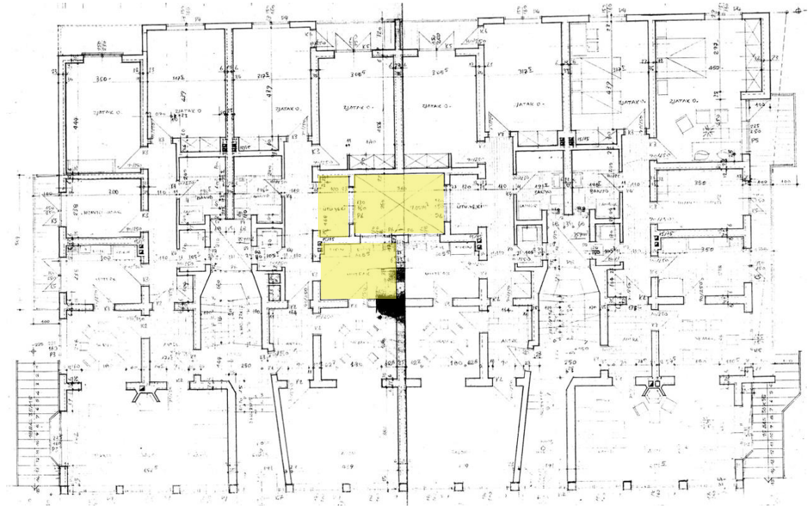
Şekil 5.57. 1962 Tekdal Apartmanı Zemin Kat Planı. Kaynak: Sivil Mimari Bellek Ankara 1930-1980 Projesi Arşivi, URL 22 Erişim:03.05.2025
