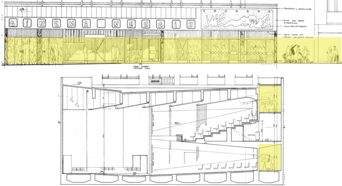
Şekil 5.113. 1965 Başkent Apartmanı Mimari Çizim Temsilleri. Kaynak: Sivil Mimari Bellek Ankara 1930-1980 Projesi Arşivi, URL 22 Erişim:03.05.2025
