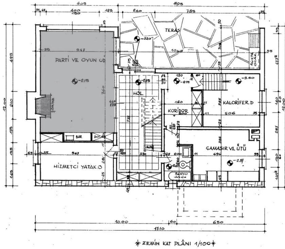
Şekil 5.53. 1960 Turhan Türker Evi Birinci Kat Planı. Kaynak: Sivil Mimari Bellek Ankara 1930-1980 Projesi Arşivi, URL 22 Erişim:03.05.2025
