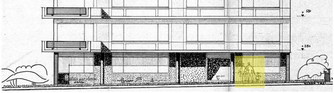
Şekil 5.78. 1956 Übeyde Elli Apartmanı Ön Cephe. Kaynak: Sivil Mimari Bellek Ankara 1930-1980 Projesi Arşivi, URL 22 Erişim:03.05.2025
