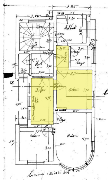
Şekil 5.23. 1930 İçöz Apartmanı Birinci Kat Planı. Kaynak: Sivil Mimari Bellek Ankara 1930-1980 Projesi Arşivi, URL 22 Erişim:03.05.2025
