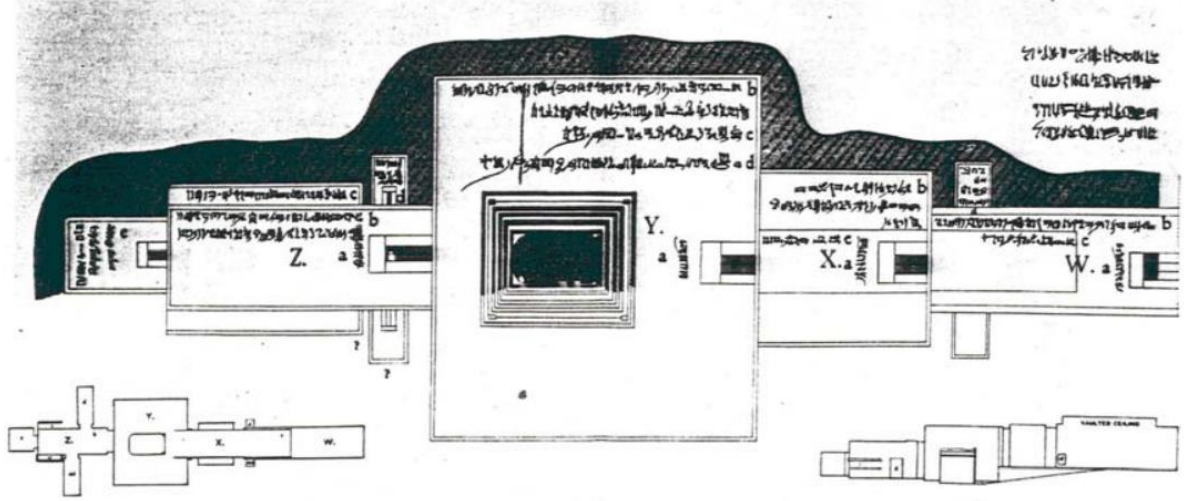
Şekil 5.1. IV Ramses'in Mezar Planı, Papirüs Kağıdına Çizim. Kaynak: Halse, 1960, akt. Gürer ve Yücel, 2005
