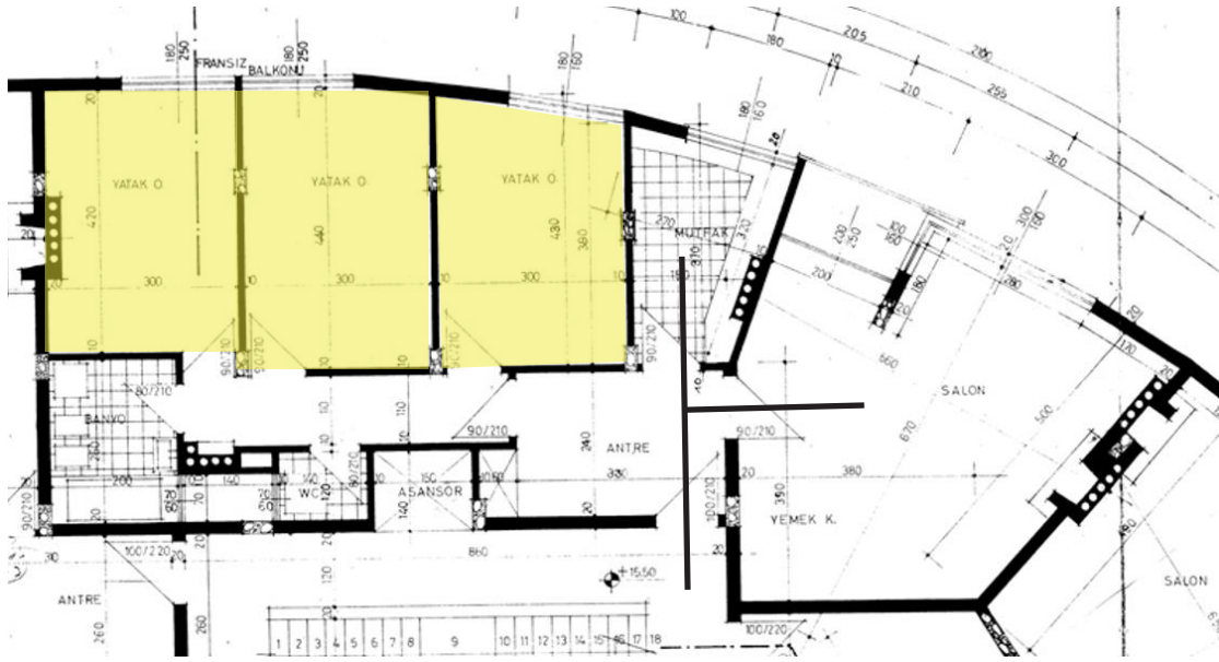
Şekil 5.61. 1964 Çırağan Apartmanı Normal Kat Planı, Daire. Kaynak: Sivil Mimari Bellek Ankara 1930-1980 Projesi Arşivi, URL 22 Erişim:03.05.2025
