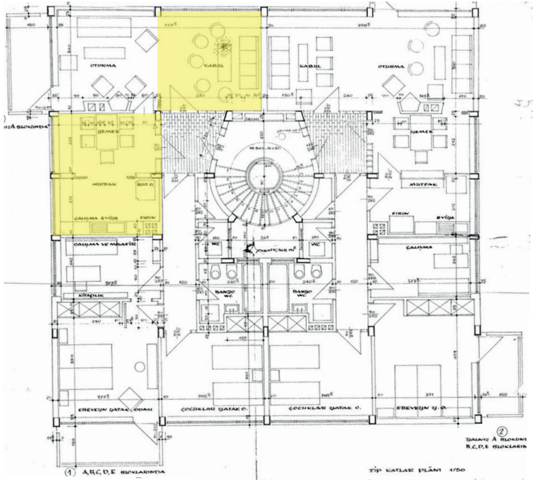
Şekil 5.50. 1960 Basın Sitesi I. Tip Katlar Planı. Kaynak: Sivil Mimari Bellek Ankara 1930-1980 Projesi Arşivi, URL 22 Erişim:03.05.2025
