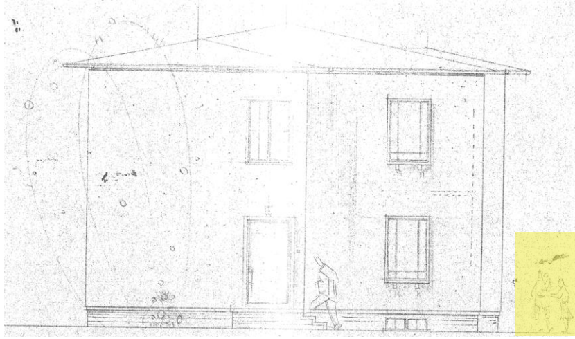
Şekil 5.69. 1952 Kavacık Ucuz Subayevleri Ön Cephe Görünüş. Kaynak: Sivil Mimari Bellek Ankara 1930-1980 Projesi Arşivi, URL 22 Erişim:03.05.2025
