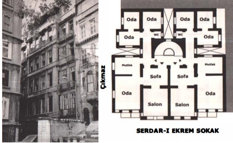
Şekil 4.9. Dikeos Apartmanları Plan Şemaları, Kaynak: Apartman, Galata'da Yeni Bir Konut Tipi, s.412-413 Erişim:10.05.2025
