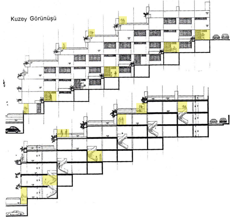
Şekil 5.123. 1981 Teras Ev Kuzey Görünüş. Kaynak: Sivil Mimari Bellek Ankara 1930-1980 Projesi Arşivi, URL 22 Erişim:03.05.2025
