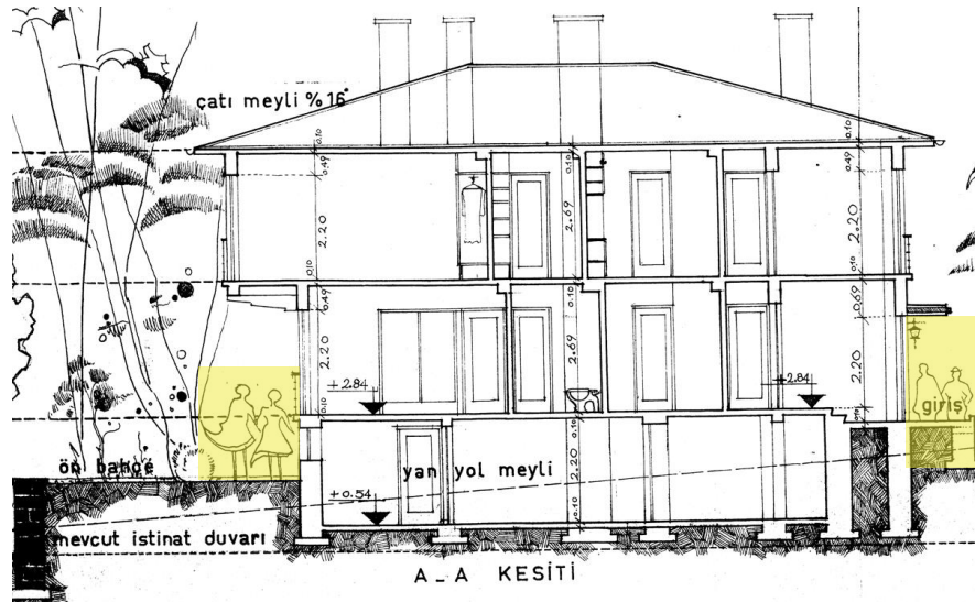
Şekil 5.114. 1966 İrfan Küçük Apartmanı A.A Kesit. Kaynak: Sivil Mimari Bellek Ankara 1930-1980 Projesi Arşivi, URL 22 Erişim:03.05.2025
