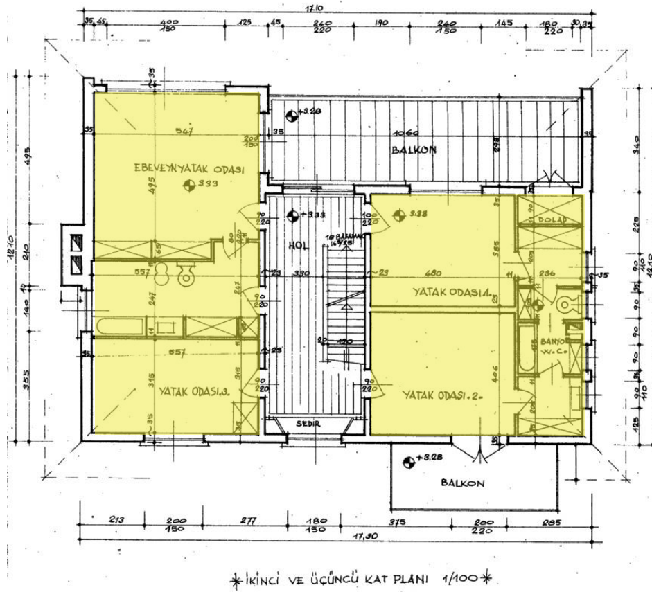
Şekil 5.54. 1960 Turhan Türker Evi İkinci ve Üçüncü Kat Planı. Kaynak: Sivil Mimari Bellek Ankara 1930-1980 Projesi Arşivi, URL 22 Erişim:03.05.2025
