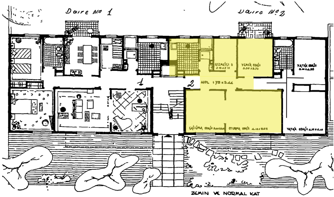
Şekil 5.38. 1955 İsrailcileri Zemin ve Normal Kat Planı. Kaynak: Sivil Mimari Bellek Ankara 1930-1980 Projesi Arşivi, URL 22 Erişim:03.05.2025
