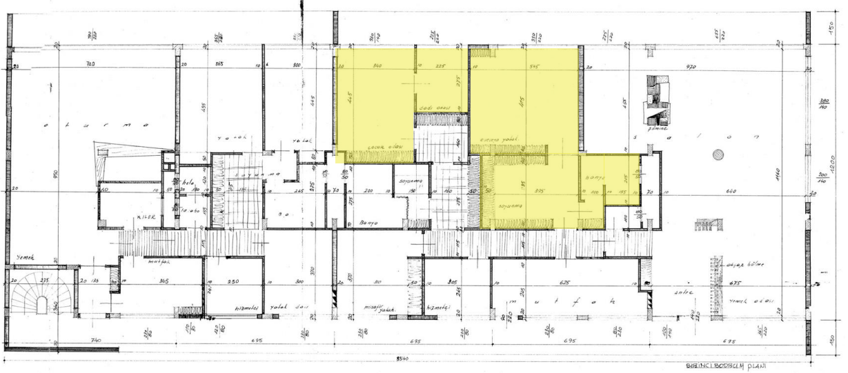
Şekil 5.48. 1958 Cinnah 19 Birinci Bodrum Kat Planı. Kaynak: Sivil Mimari Bellek Ankara 1930-1980 Projesi Arşivi, URL 22 Erişim:03.05.2025
