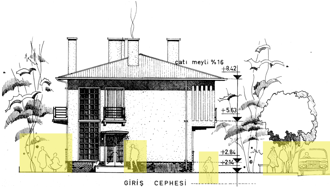
Şekil 5.115. 1966 İrfan Küçük Apartmanı Giriş Cephesi Görünüş. Kaynak: Sivil Mimari Bellek Ankara 1930-1980 Projesi Arşivi, URL 22 Erişim:03.05.2025
