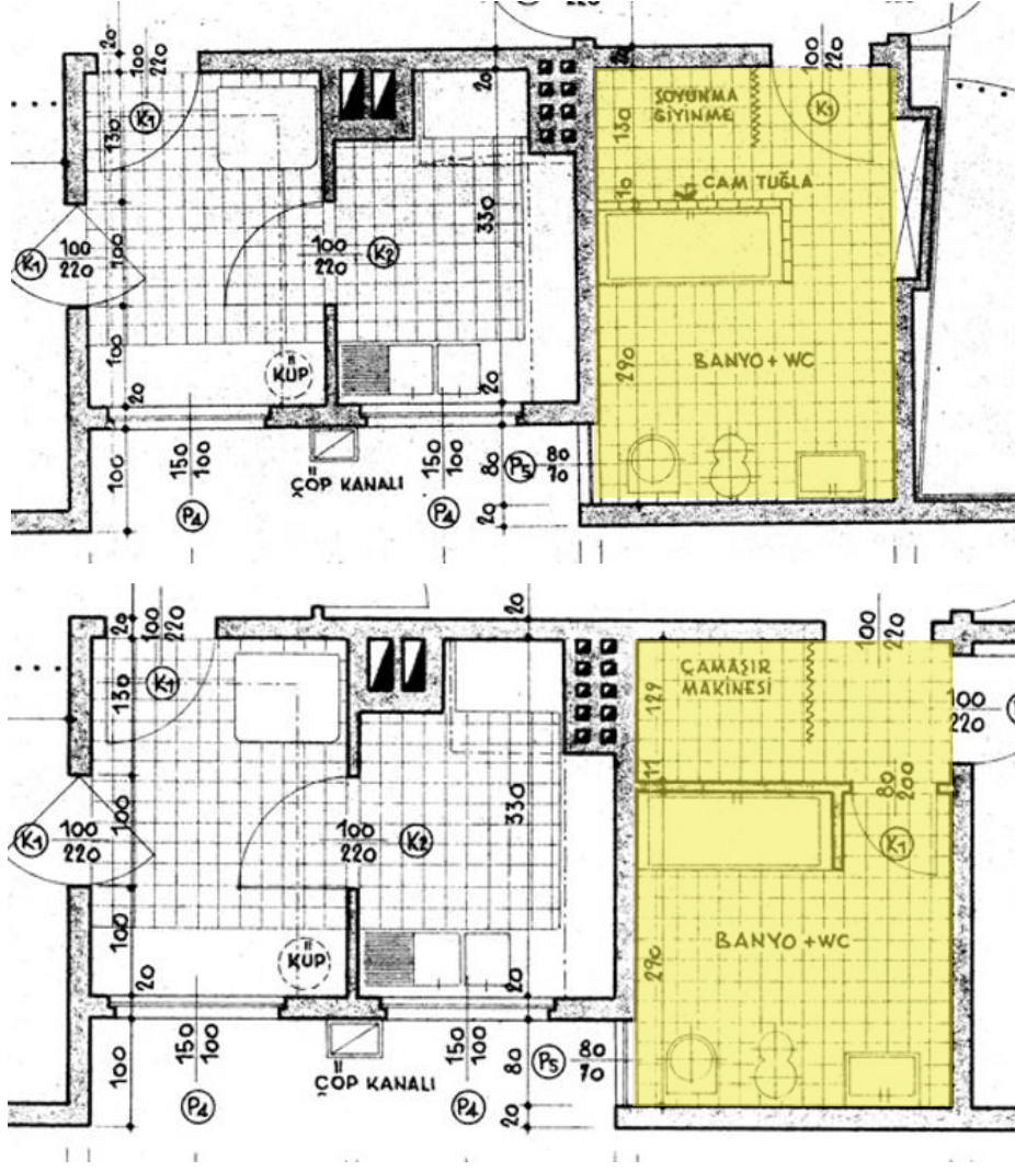
Şekil 5.44. 1957 Sönmez Apartmanı’nda Islak Hacimlerin Biçimlenmesi. Kaynak: Sivil Mimari Bellek Ankara 1930-1980 Projesi Arşivi, URL 22 Erişim:03.05.2025
