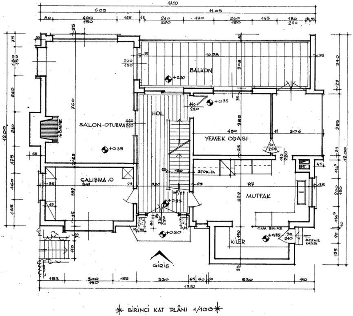
Şekil 5.52. 1960 Turhan Türker Evi Zemin Kat Planı. Kaynak: Sivil Mimari Bellek Ankara 1930-1980 Projesi Arşivi, URL 22 Erişim:03.05.2025
