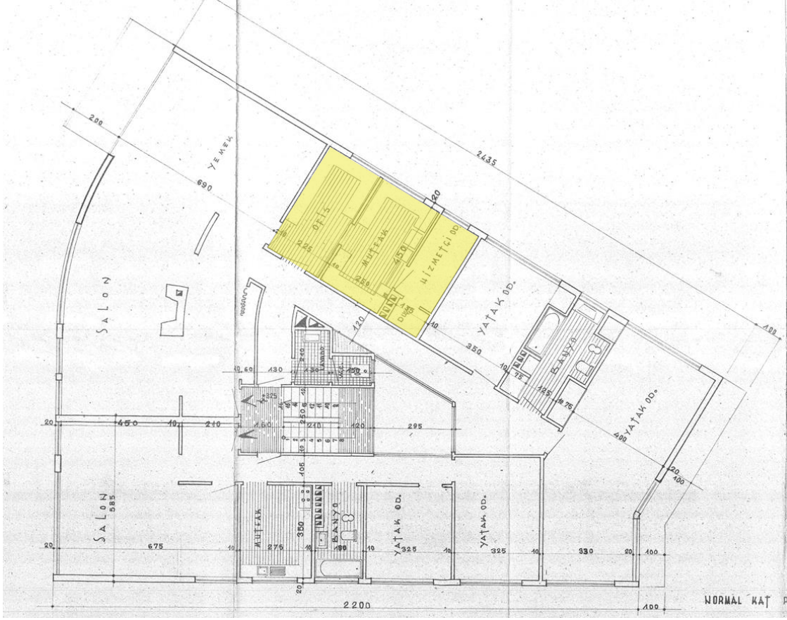
Şekil 5.42. 1956 Übeyde Elli Apartmanı Normal Kat Planı. Kaynak: Sivil Mimari Bellek Ankara 1930-1980 Projesi Arşivi, URL 22 Erişim:03.05.2025
