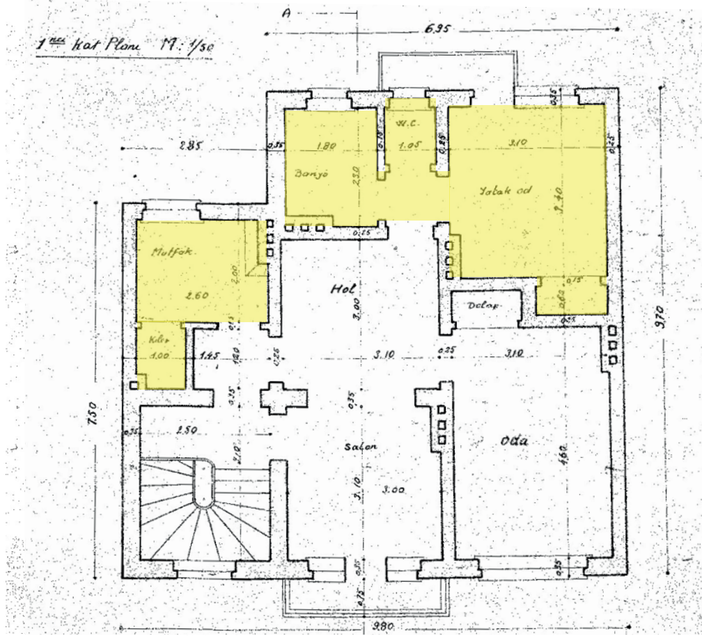
Şekil 5.28. 1947 Cemal Poyrazoğlu Apartmanı 1.Kat Planı. Kaynak: Sivil Mimari Bellek Ankara 1930-1980 Projesi Arşivi, URL 22 Erişim:03.05.2025
