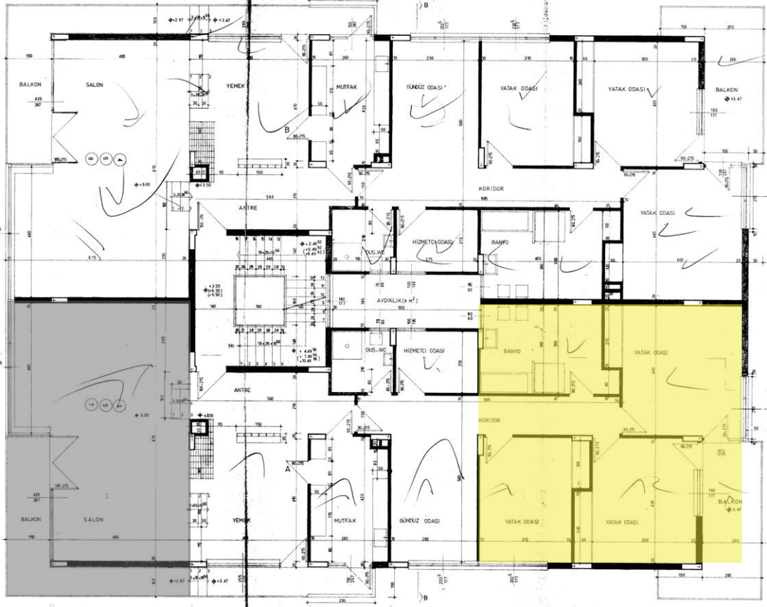
Şekil 5.63. 1965 İbrahim Ethem Kavşit Apartmanı. Kaynak: Sivil Mimari Bellek Ankara 1930-1980 Projesi Arşivi, URL 22 Erişim:03.05.2025
