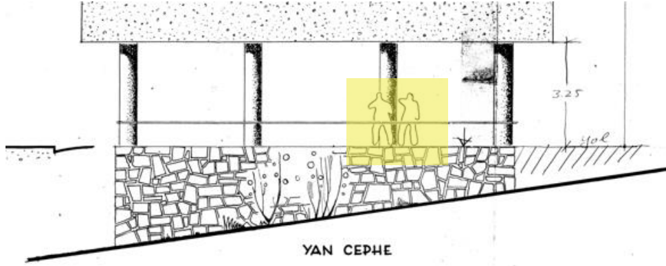
Şekil 5.89. 1957 Mintrak Apartmanı Yan Cephe Görünüş. Kaynak: Sivil Mimari Bellek Ankara 1930-1980 Projesi Arşivi, URL 22 Erişim:03.05.2025
