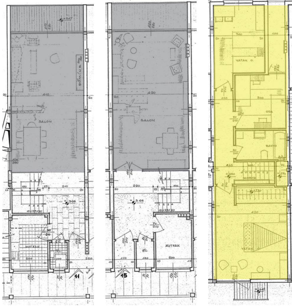
Şekil 5.58. 1962 Öz-Ok Apartmanı Dubleks Daire Birinci ve İkinci Kat Planları. Kaynak: Sivil Mimari Bellek Ankara 1930-1980 Projesi Arşivi, URL 22 Erişim:03.05.2025
