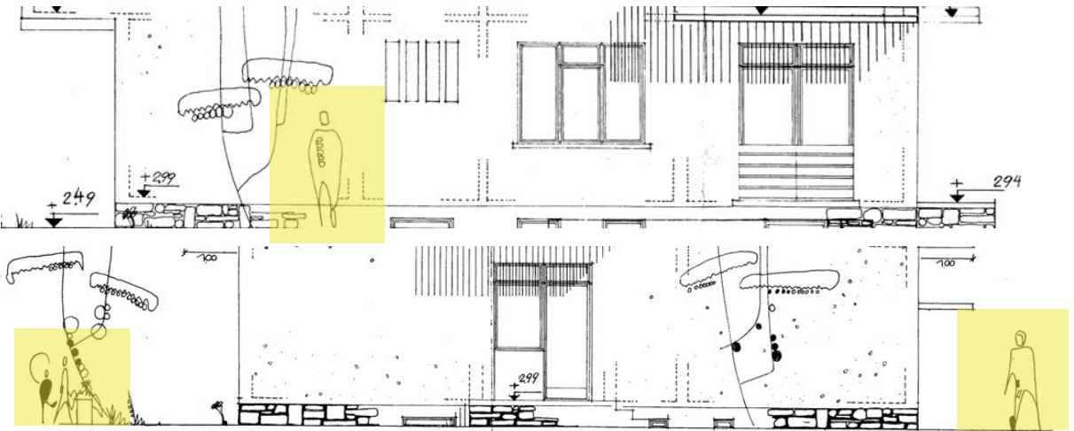
Şekil 5.108. 1963 İlkadım 22 Yan Cephe ve Arka Cephe Görünüş Çizimi. Kaynak: Sivil Mimari Bellek Ankara 1930-1980 Projesi Arşivi, URL 22 Erişim:03.05.2025
