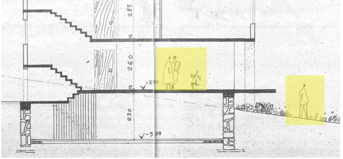
Şekil 5.75. 1956 Übeyde Elli Apartmanı A.A Kesit. Kaynak: Sivil Mimari Bellek Ankara 1930-1980 Projesi Arşivi, URL 22 Erişim:03.05.2025
