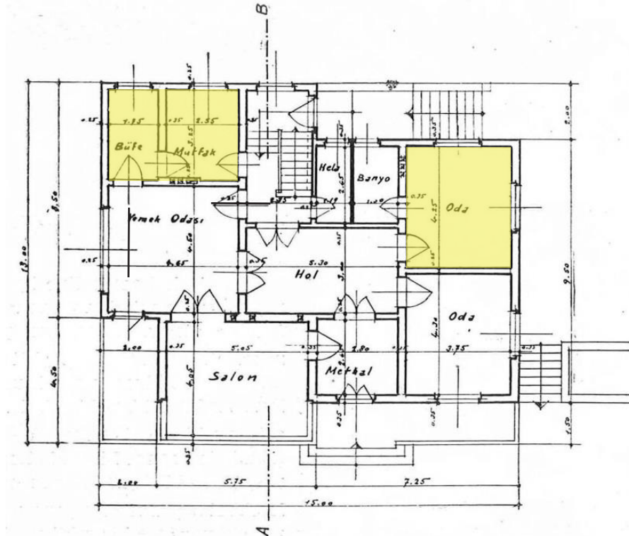
Şekil 5.25. 1932 İsmail Hakkı Bey Evi Zemin Kat Planı Kaynak: Sivil Mimari Bellek Ankara 1930-1980
