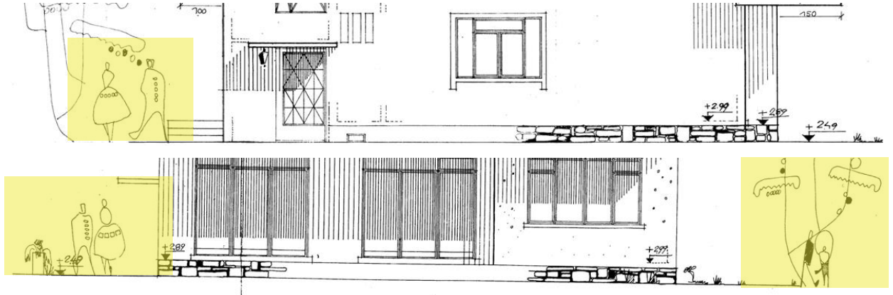
Şekil 5.109. 1963 İlkadım 22 Giriş Cephe ve Ön Cephe Görünüş Çizimi. Kaynak: Sivil Mimari Bellek Ankara 1930-1980 Projesi Arşivi, URL 22 Erişim:03.05.2025
