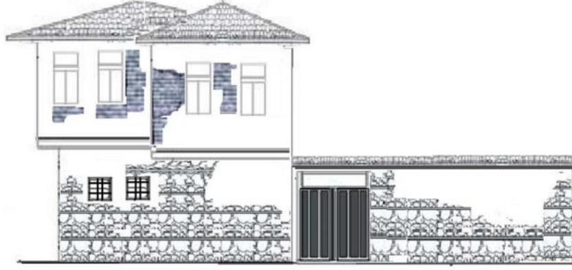
Şekil 4.4. Selahattin Taştekin Evi'nin Yol Cephesi Çizimi Kaynak: Demirci, 2021 s.103
