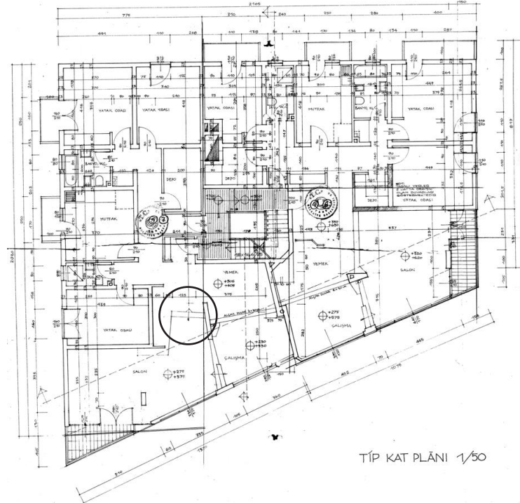
Şekil 5.60. 1963 Kader 1 Tip Kat Planı. Kaynak: Sivil Mimari Bellek Ankara 1930-1980 Projesi Arşivi, URL 22 Erişim:03.05.2025
