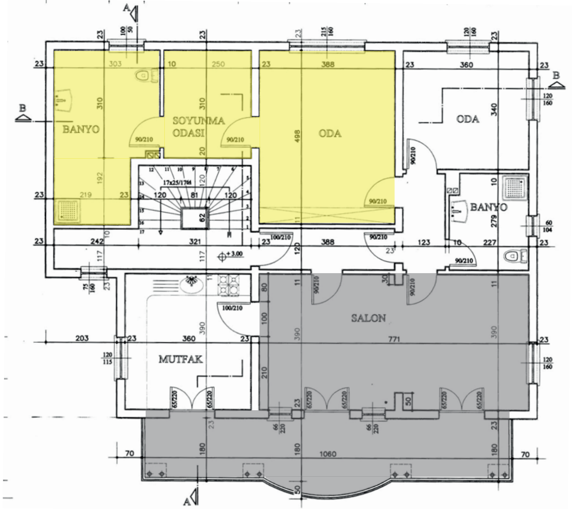
Şekil 5.33. 1951 14 Mayıs Evleri, Tip 2, İran Caddesi No 31. 1.Normal Kat Planı. Kaynak: Sivil Mimari Bellek Ankara 1930-1980 Projesi Arşivi, URL 22 Erişim:03.05.2025
