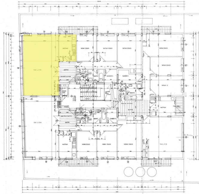
Şekil 5.65. 1965 Başkent Apartmanı Tip Kat Planı. Kaynak: Sivil Mimari Bellek Ankara 1930-1980 Projesi Arşivi, URL 22 Erişim:03.05.2025
