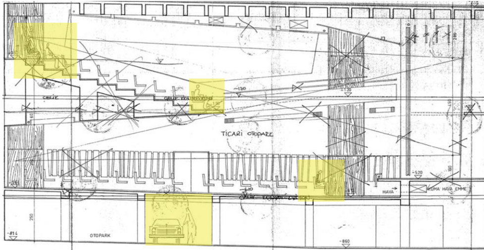
Şekil 5.120. 1969 Talip Apartmanı Kesit Çizimi Talip Sineması. Kaynak: Sivil Mimari Bellek Ankara 1930-1980 Projesi Arşivi, URL 22 Erişim:03.05.2025
