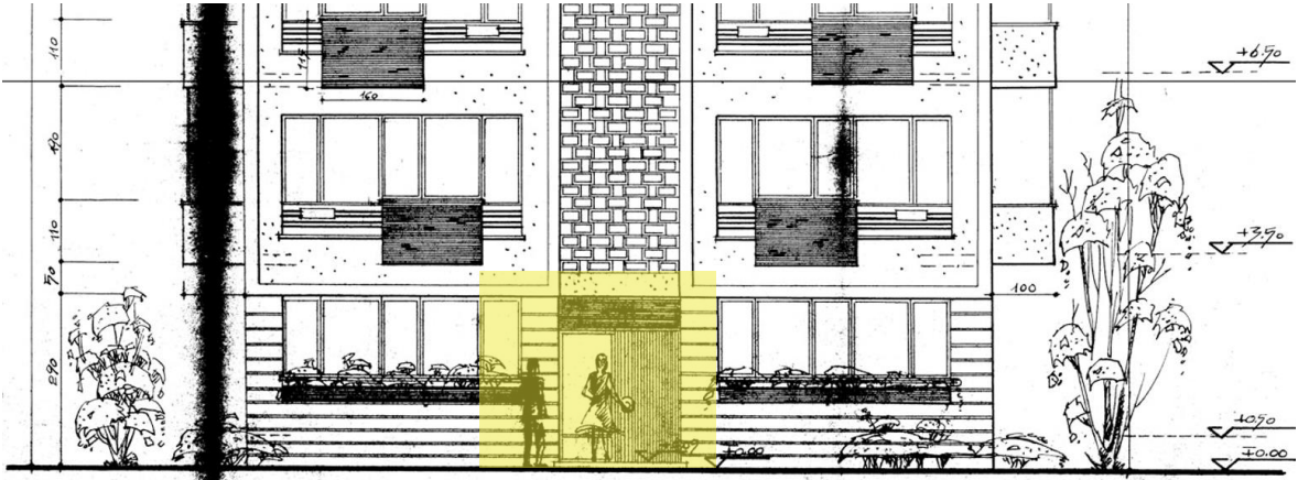
Şekil 5.112. 1964 Eren Apartmanı Görünüş Çizimi. Kaynak: Sivil Mimari Bellek Ankara 1930-1980 Projesi Arşivi, URL 22 Erişim:03.05.2025
