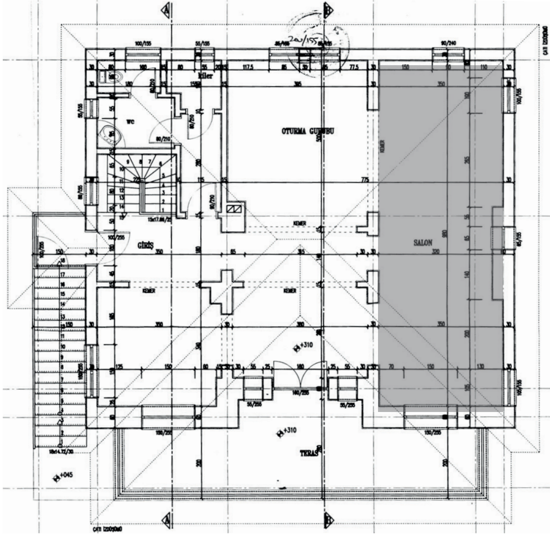
Şekil 5.31. 1951 14 Mayıs Evleri, Tip 1, Budak Sokak No 1, 1. Kat Planı. Kaynak: Sivil Mimari Bellek Ankara 1930-1980 Projesi Arşivi, URL 22 Erişim:03.05.2025
