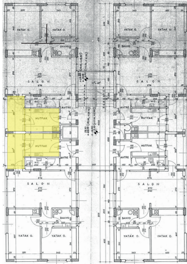
Şekil 5.55. 1961 Güneş Sitesi Normal Kat Planı. Kaynak: Sivil Mimari Bellek Ankara 1930-1980
