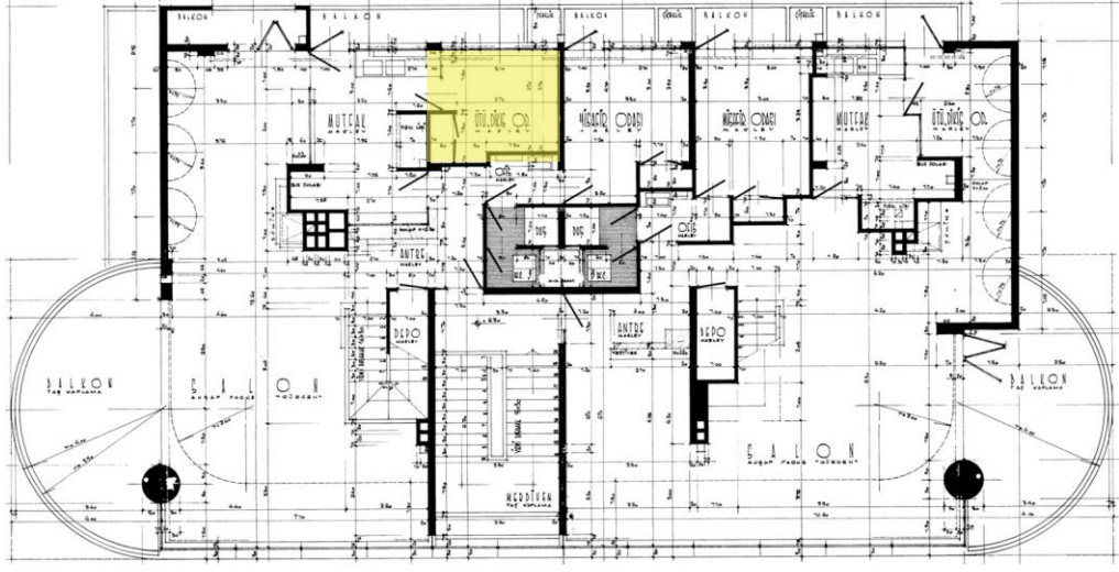
Şekil 5.66. 1968 Özkanlar Evi İkinci Kat Planı. Kaynak: Sivil Mimari Bellek Ankara 1930-1980 Projesi Arşivi, URL 22 Erişim:03.05.2025
