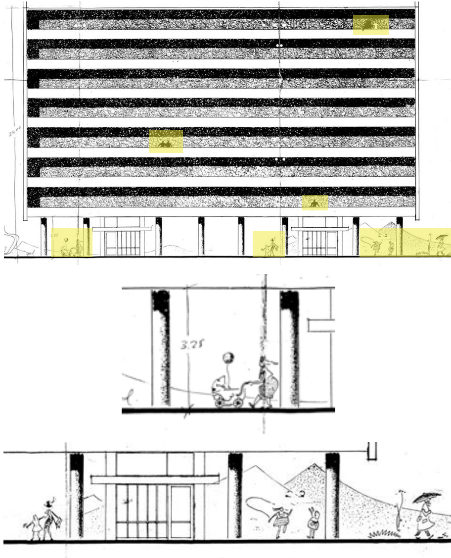
Şekil 5.90. 1957 Mintrak Apartmanı Ön Cephe Görünüş. Kaynak: Sivil Mimari Bellek Ankara 1930-1980 Projesi Arşivi, URL 22 Erişim:03.05.2025
