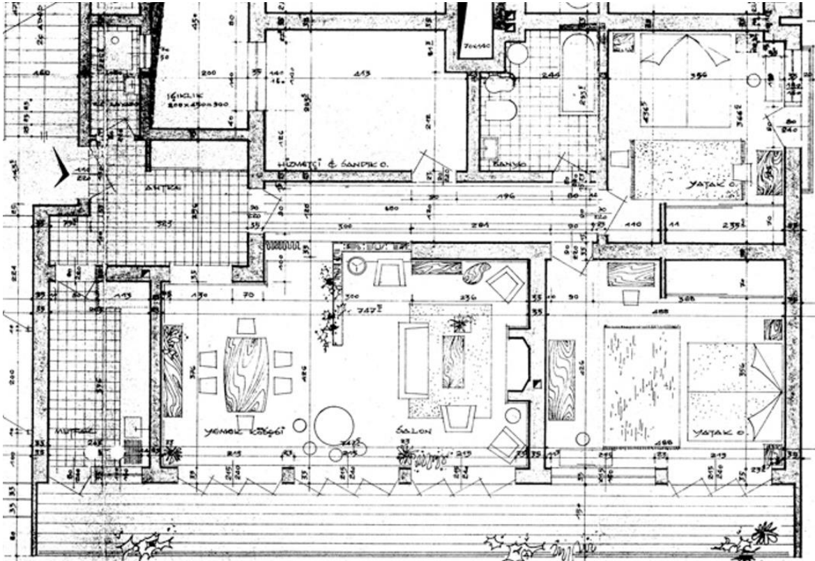
Şekil 5.51. 1960 İpek Apartmanı Zemin Kat Planı. Kaynak: Sivil Mimari Bellek Ankara 1930-1980 Projesi Arşivi, URL 22 Erişim:03.05.2025
