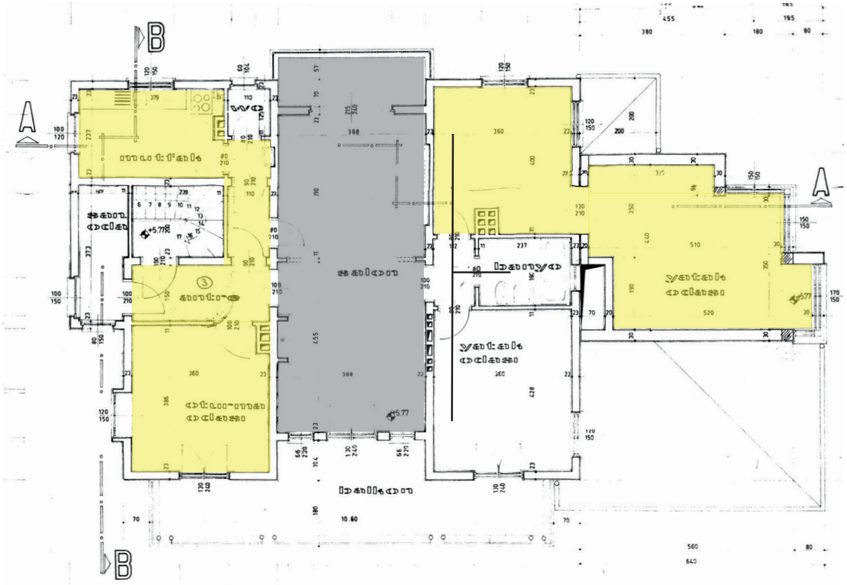
Şekil 5.32. 1951 14 Mayıs Evleri, Tip 2, Arjantin Caddesi No 2. 2.Kat Planı. Kaynak: Sivil Mimari Bellek Ankara 1930-1980 Projesi Arşivi, URL 22 Erişim:03.05.2025
