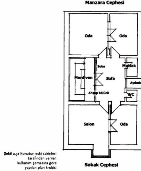
Şekil 4.8. Konut Plan Şeması, Kaynak: Apartman, Galata'da Yeni Bir Konut Tipi, s.141 Erişim:10.05.2025
