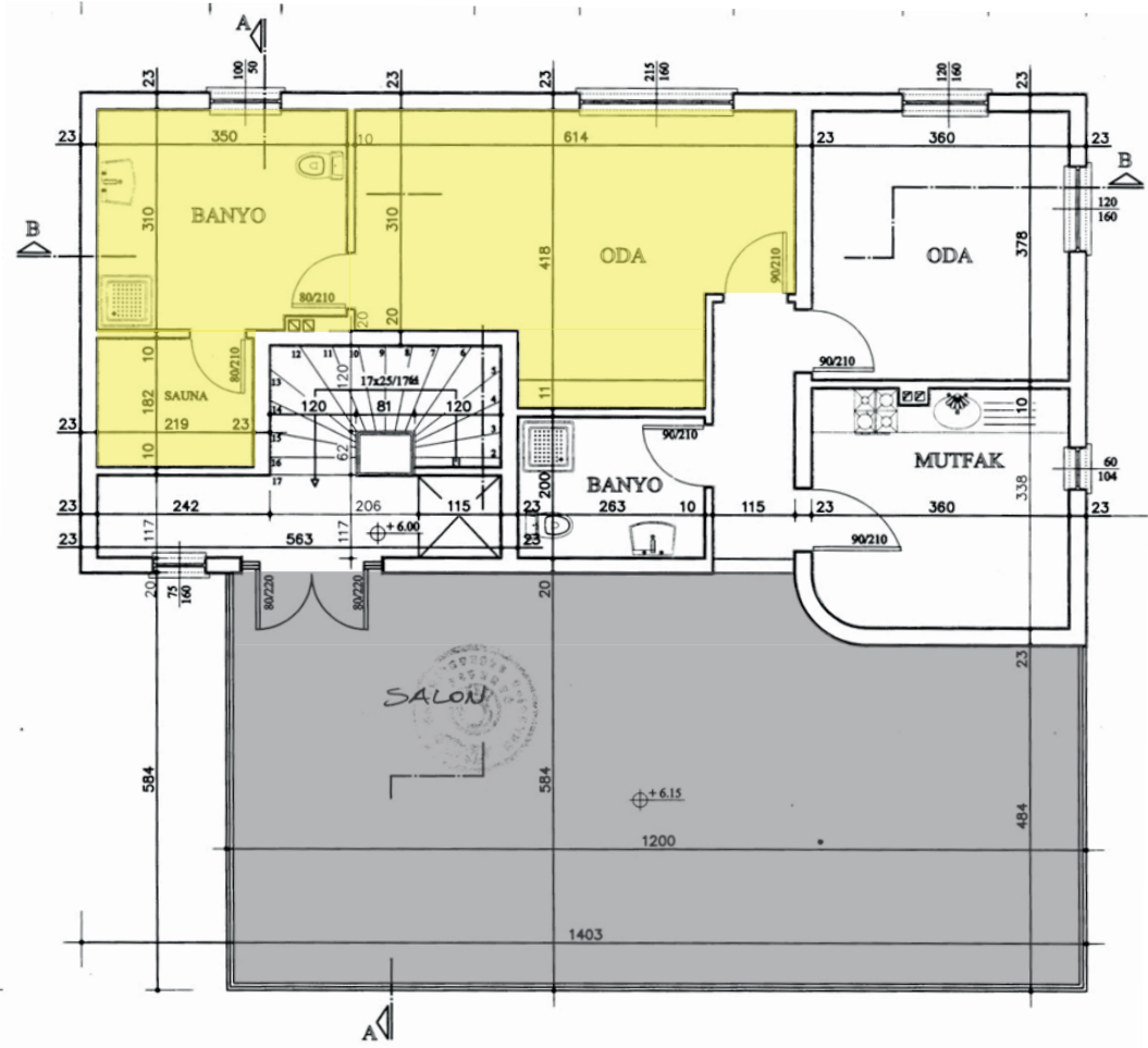
Şekil 5.34. 1951 14 Mayıs Evleri, Tip 2, İran Caddesi No 31. 2.Normal Kat Planı. Kaynak: Sivil Mimari Bellek Ankara 1930-1980 Projesi Arşivi, URL 22 Erişim:03.05.2025
