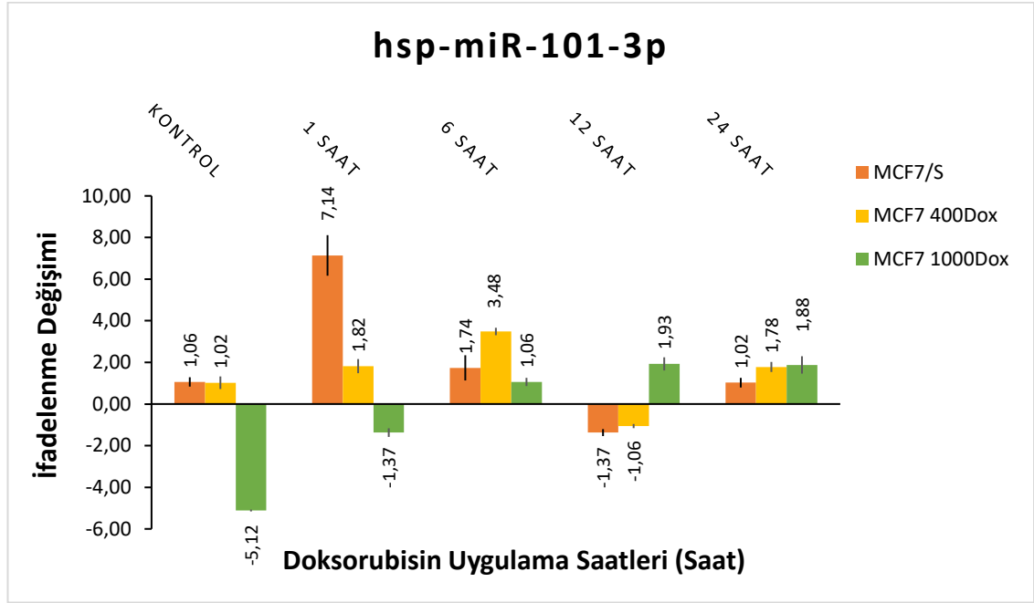
Şekil 24: Hsp-miR-101'in ifadenme değişimi grafiği.
