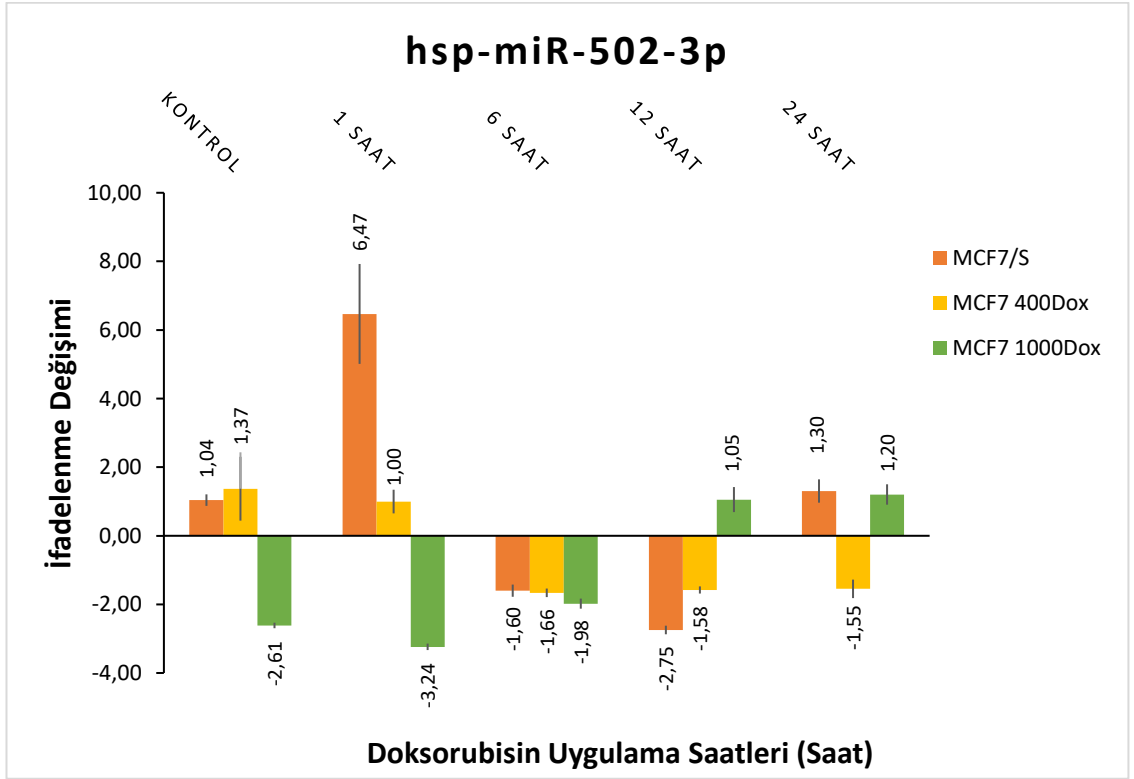
Şekil 27: Hsp-miR-502-3p ifadeleme değişimi.
