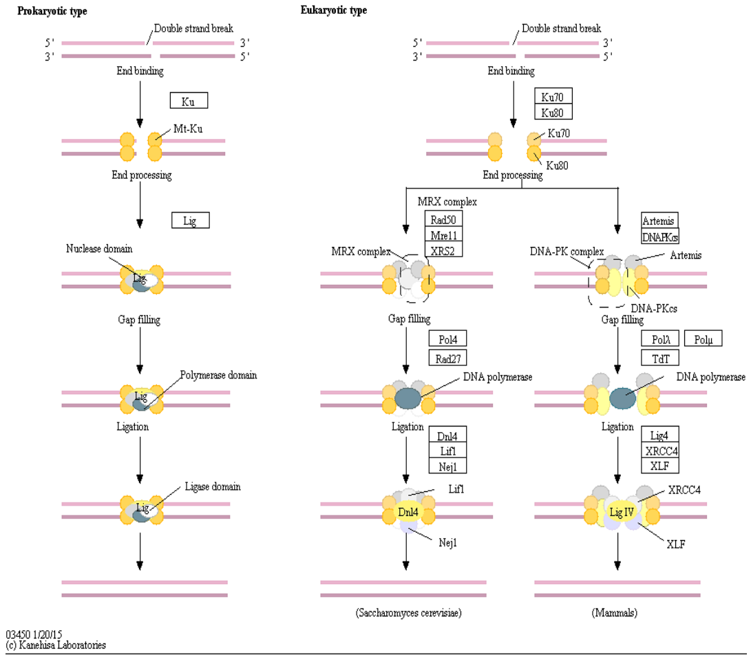
Şekil 7: NHEJ mekanizması (Ekim 2018, KEGG)
