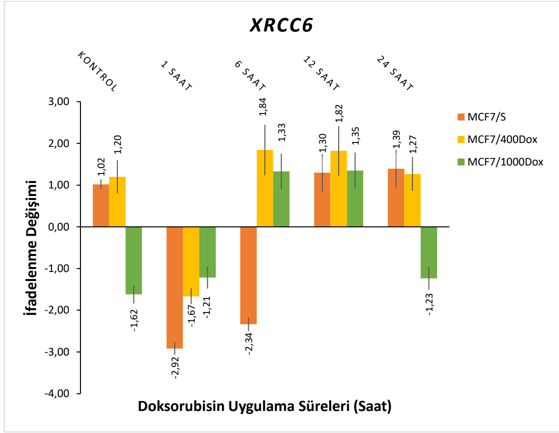
Şekil 18: XRCC6 gen ifadenme analizleri.
