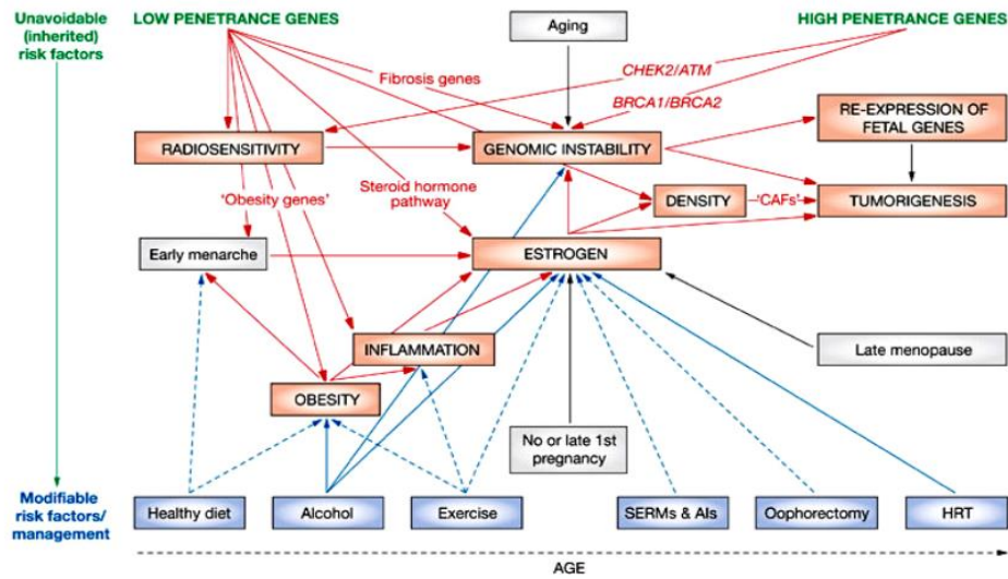
Şekil 1: Meme kanseri ile ilişkili olan faktörler (17).
