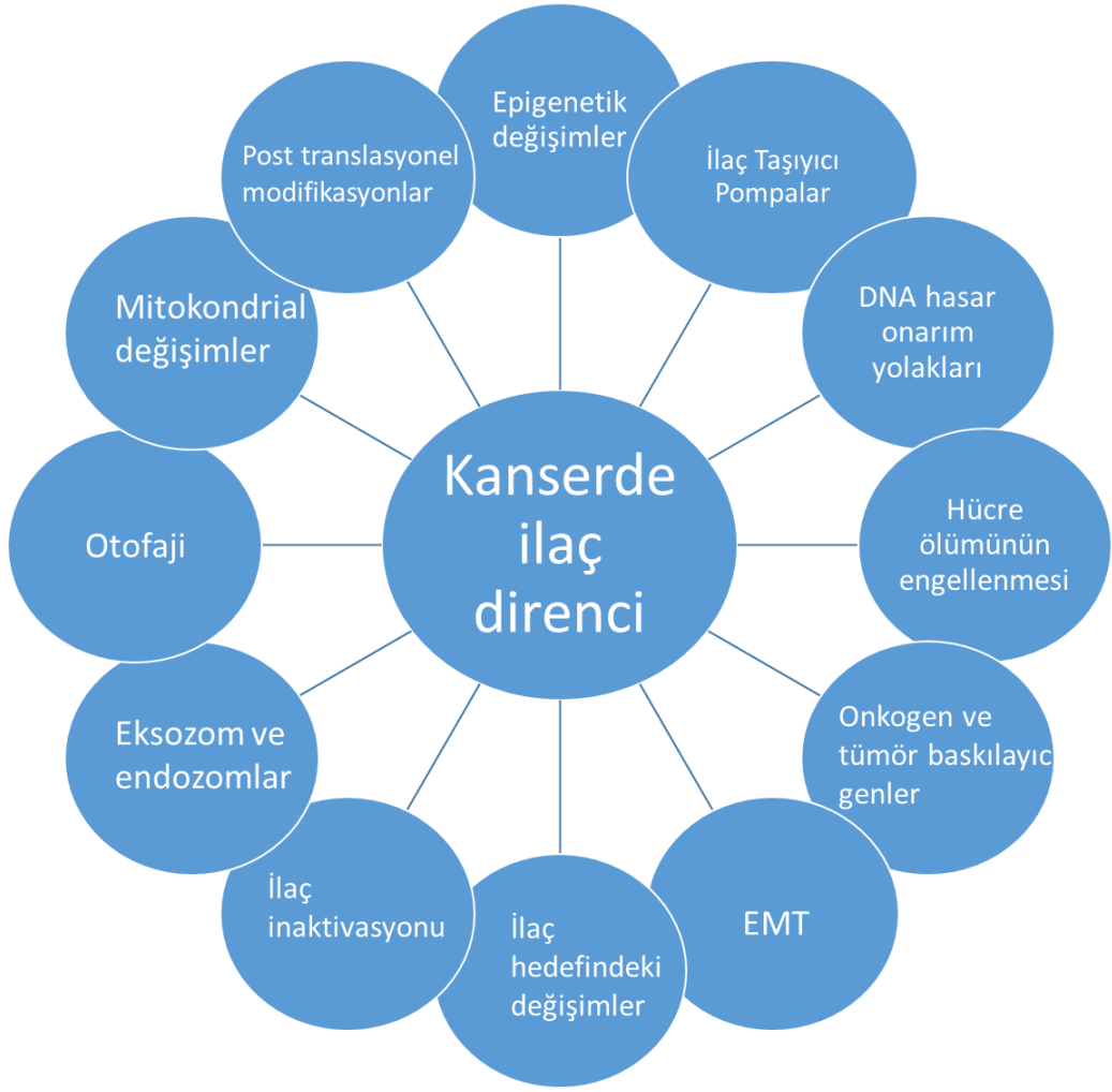
Şekil 4: Doğrudan veya dolaylı olarak ilaç direnci oluşumuna neden olan mekanizmalar (39, 40)
