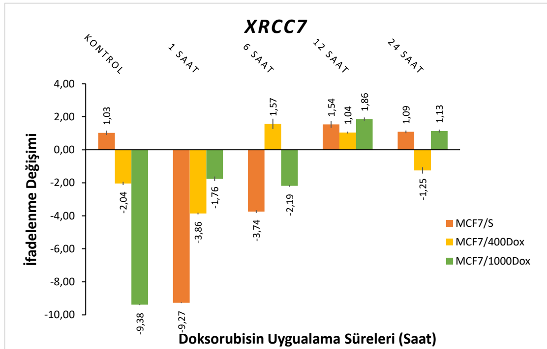
Şekil 19: XRCC7 gen ifadenme analizleri.
